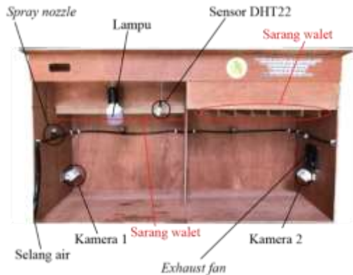
Gambar 11. Prototipe Rumah Sarang Burung Walet
