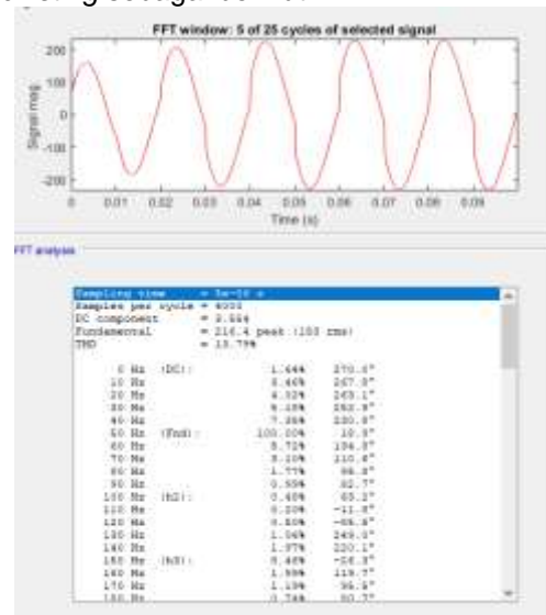
Gambar 3: Hasil simulasi phasa R kondisi existing
