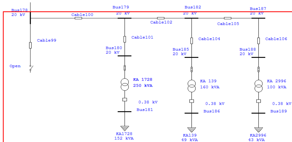
Gambar 1 Pemodelan Jaringan Distribusi 20 KV Penyulang Kerobokan pada Program ETAP Power Station
