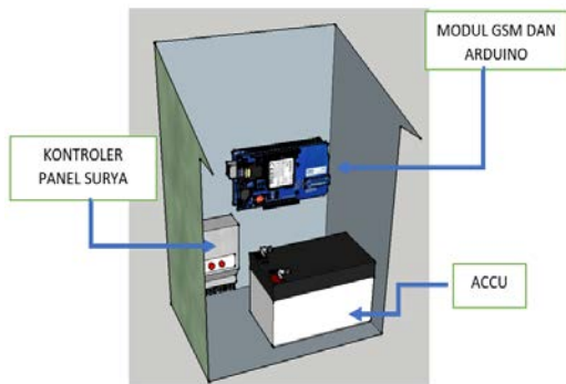
Gambar 8. Desain 3D Perangkat 1
