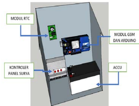
Gambar 9. Desain 3D Perangkat 2
