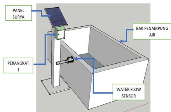
Gambar 7. Desain Bak Penampungan
