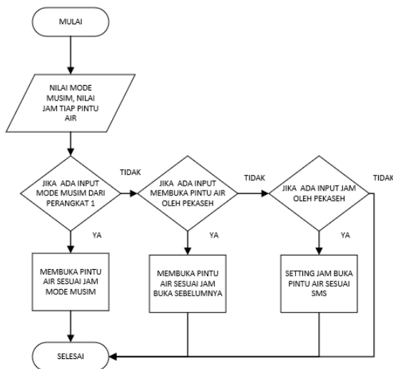
Gambar 11. Diagram Alir Perangkat 2
