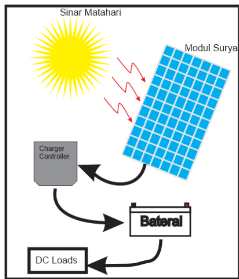
Gambar 3. Proses penggunaan Panel Surya
