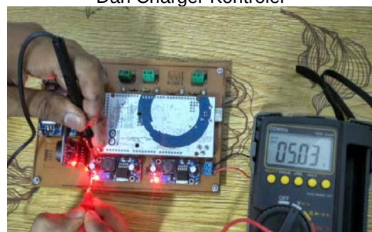
Gambar 13. Pengukuran Tegangan Input Rangkaian
