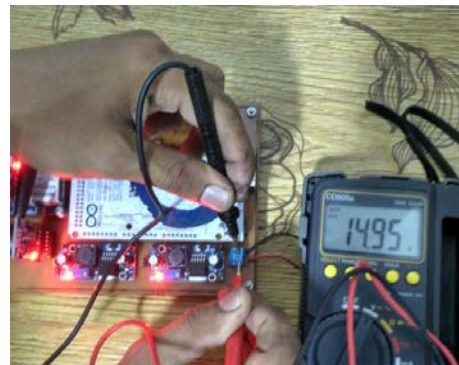
Gambar 12. Pengukuran Tegangan Input Dari Charger Kontroler
