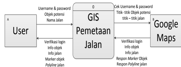
Gambar 2 Diagram Konteks
