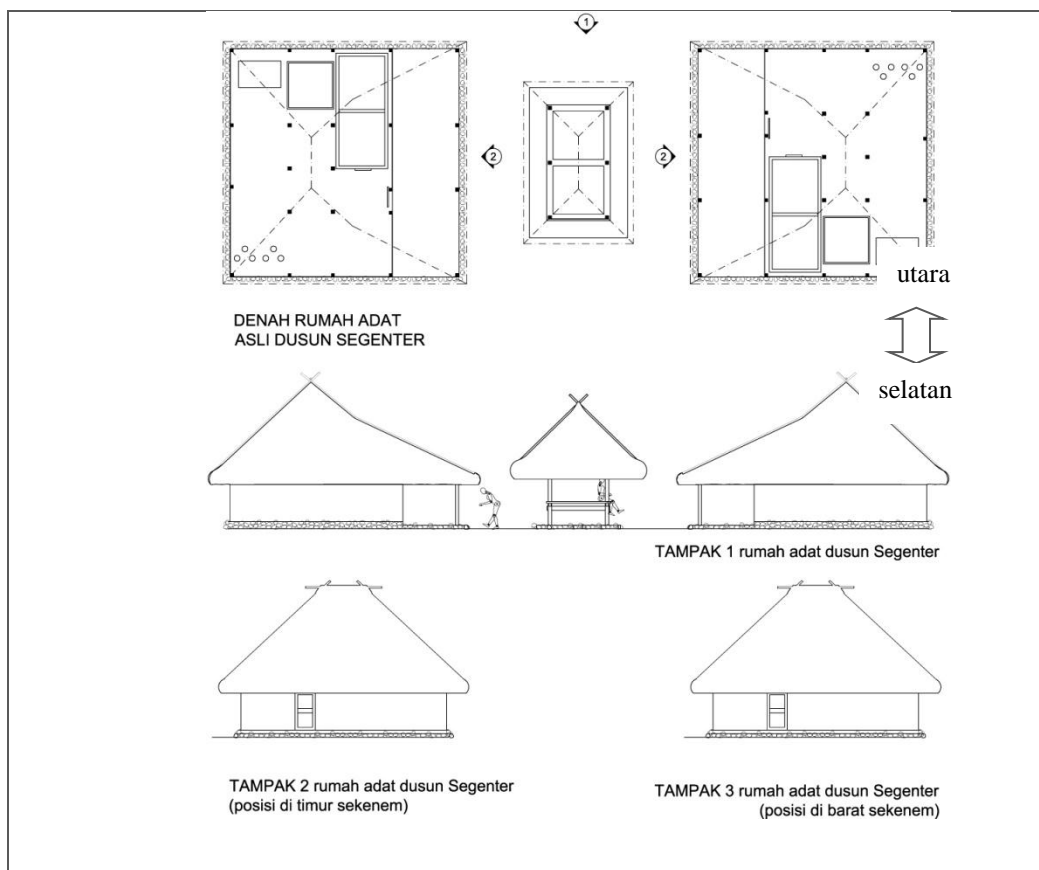
Gambar 9. Tampak bangunan rumah adat Dusun Segenter
