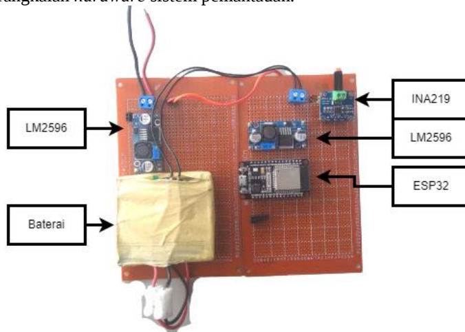
Gambar 7: Rangkaian Komponen Sistem
