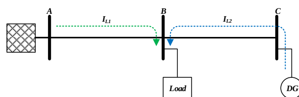
Gambar 2 : Aliran Daya pada jaringan distribusi yang tersambung dengan DG
