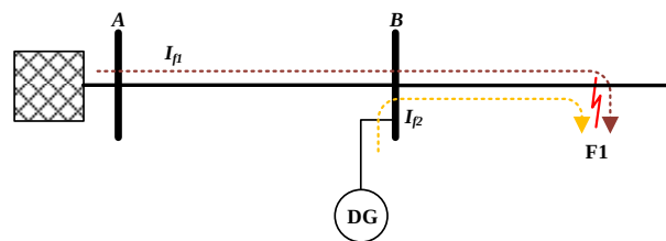
Gambar 1 : Gangguan hubung singkat pada jaringan distribusi yang tersambung dengan DG
