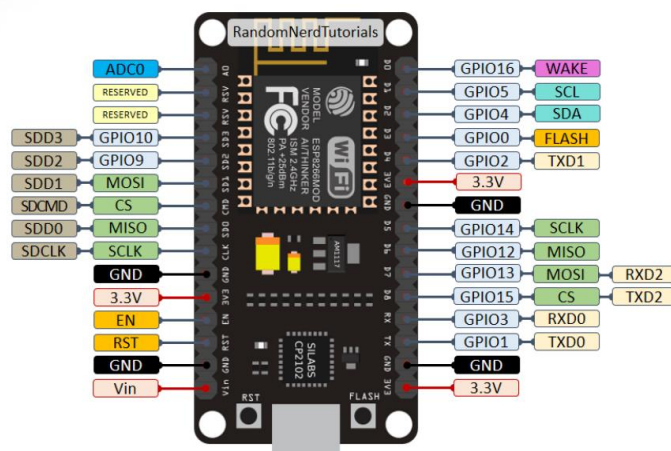
Gambar 1. Nodemcu 8266
