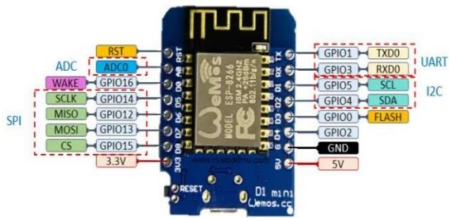
Gambar 2. Wemos D1 Mini
