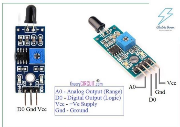
Gambar 3. Sensor Api
