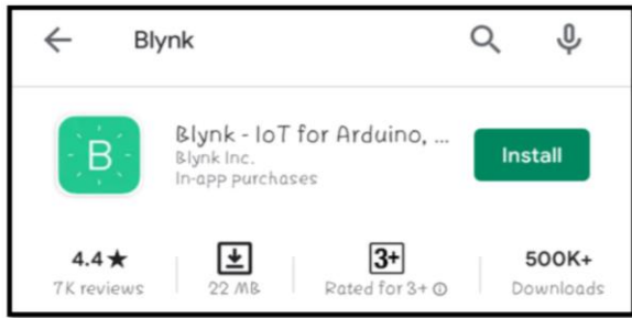
Gambar 8. Aplikasi Blynk
