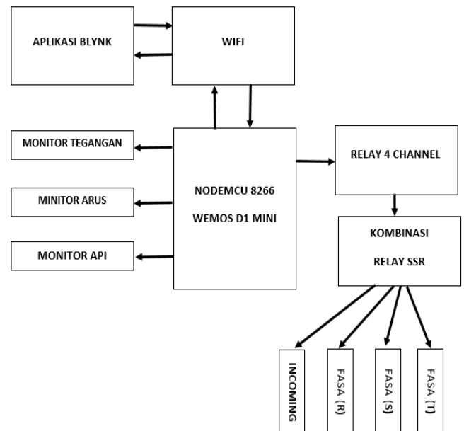
Gambar 10. Diagram Blok Proteksi Korsleting Listrik
