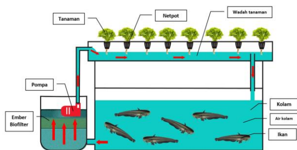
Gambar 1: Sistem Akuaponik
