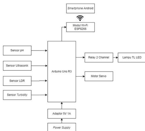
Gambar 4: Blok Sistem Hardware Akuaponik IoT
