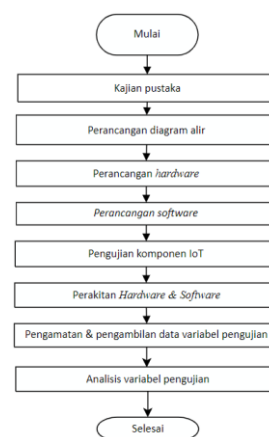
Gambar 2: Metodologi Penelitian
