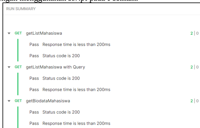
Gambar 3: Hasil Pengujian Script
