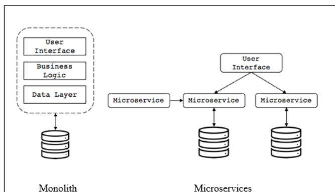
Gambar 1: Perbandingan Arsitektur Monolith dan Microservices
