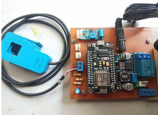
Gambar 3: realisasi pembuatan alat LANCAR
