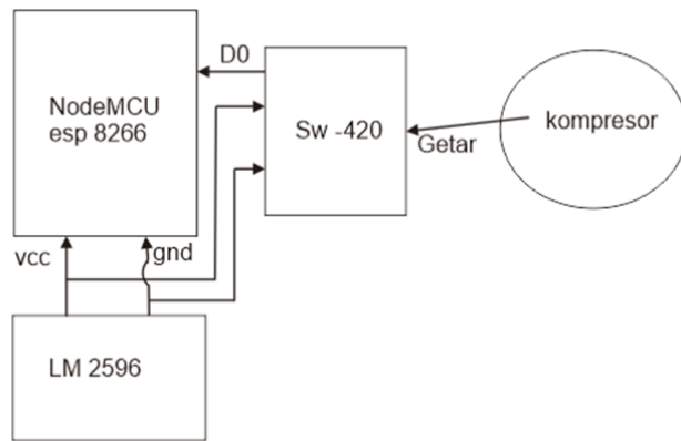
Gambar 8: Diagram Blok Pengujian Sensor Sw-420
