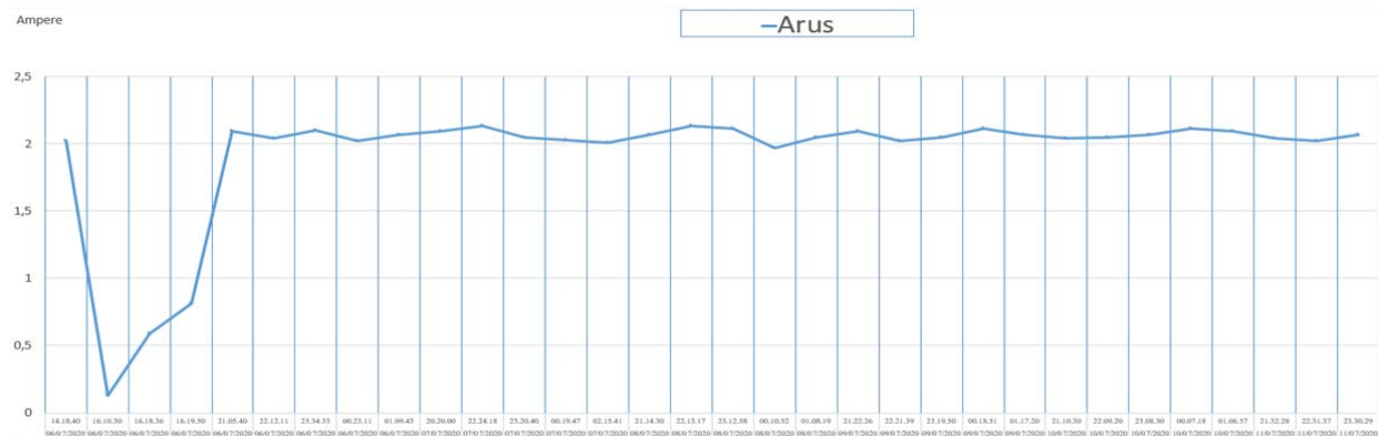
Gambar 12 : Pengujian Pada alat selama 1 minggu.
