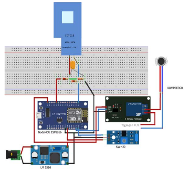
Gambar 2: wiring keseluruhan
