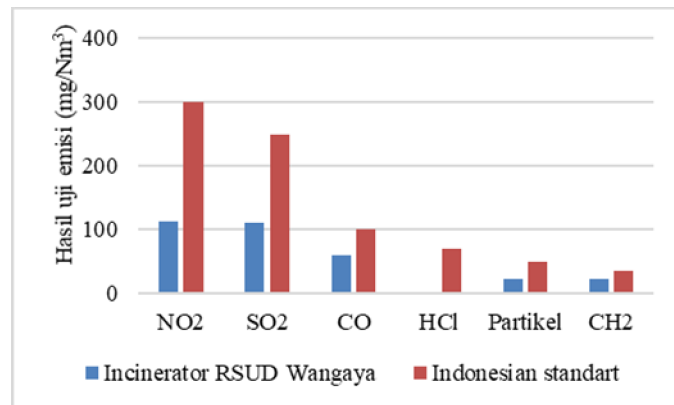
Gambar 7: Grafik hasil uji emisi incinerator
