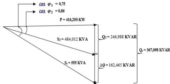
Gambar 12. Perhitungan kapasitas kapasitor bank \cos \varphi_2 = 0,86
