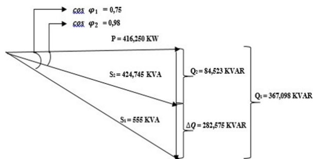
Gambar 13. Perhitungan kapasitas kapasitor bank \cos \varphi_2 = 0,98
