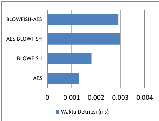
Gambar 13. Grafik Waktu Dekripsi
