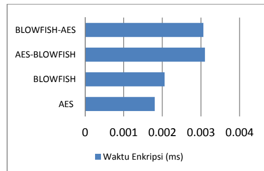
Gambar 12. Grafik Waktu Enkripsi
