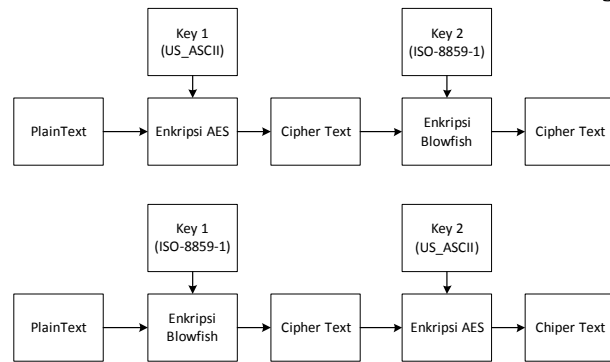
Gambar 5. proses enkripsi dengan 2 algoritma
