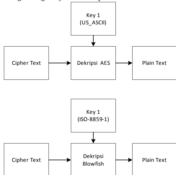
Gambar 6. proses dekripsi dengan satu algoritma
