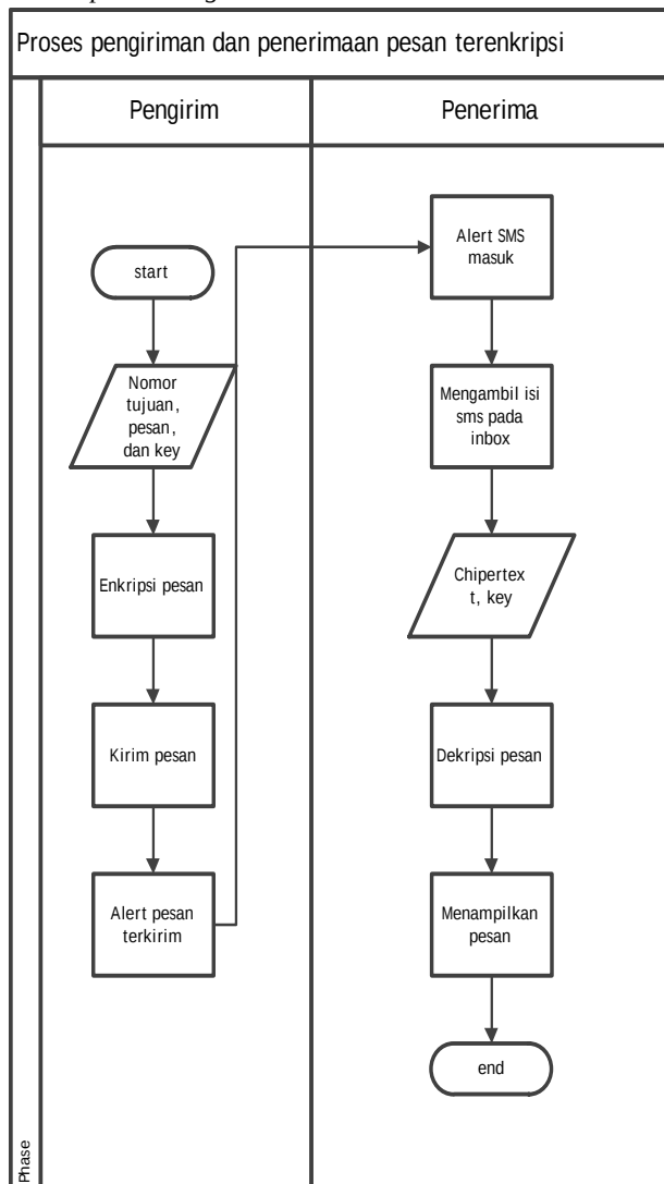
Gambar 3. Proses Pengiriman dan Penerimaan Pesan Terenkripsi
