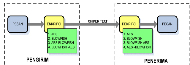
Gambar 2. Gambaran Umum Sistem
