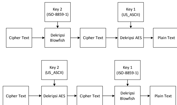
Gambar 7. proses dekripsi dengan dua algoritma
