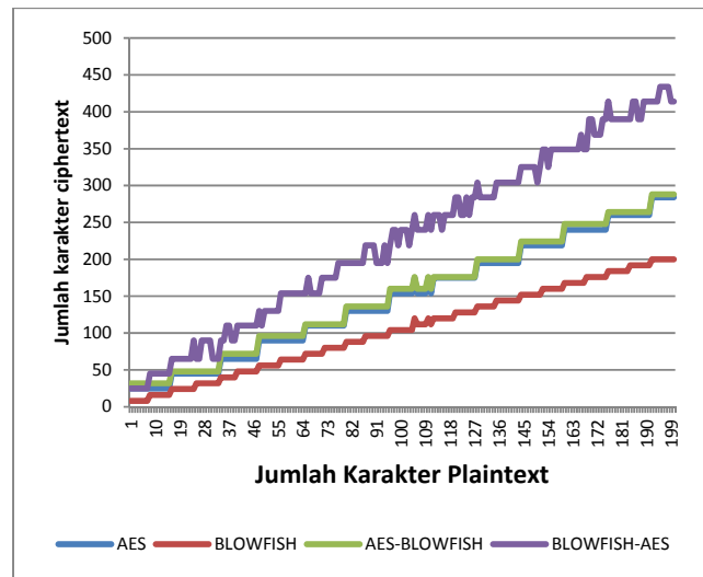
Gambar 14. Grafik Panjang Karakter
