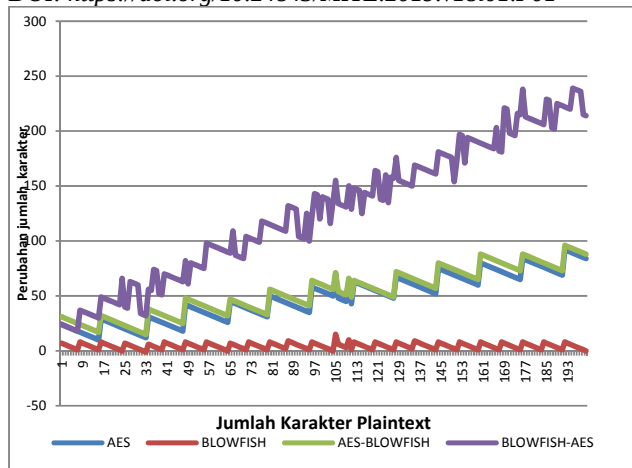
Gambar 15 Grafik Perubahan Panjang Karakter
