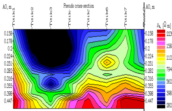
Gambar 11. Peta Isoresistivitas 2D setelah injeksi air kelima
