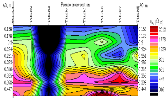
Gambar 6. Penampang isoresistivitas 2D sebelum injeksi air
