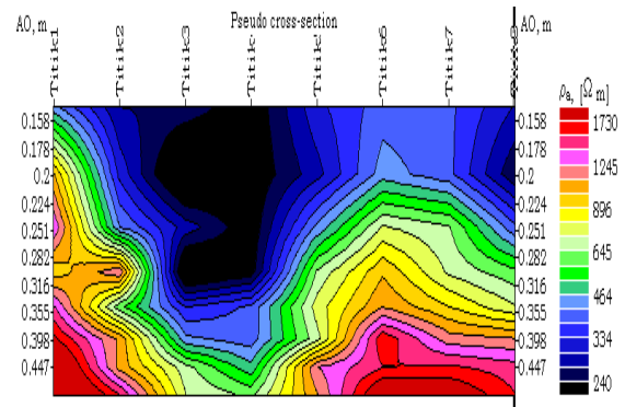
Gambar 9. Penampang Isoresistivitas 2D setelah injeksi air ketiga
