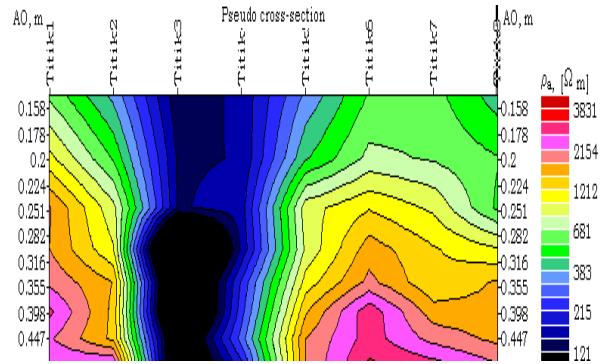
Gambar 8. Penampang Isoresistivitas 2D setelah injeksi air kedua
