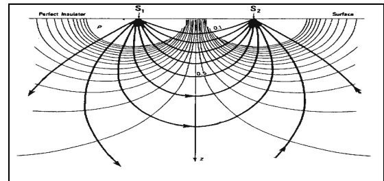
Gambar 2. Pola aliran arus dan bidang ekuipotensial antara dua elektroda arus dengan polaritas berlawanan (Bahri, 2005)
