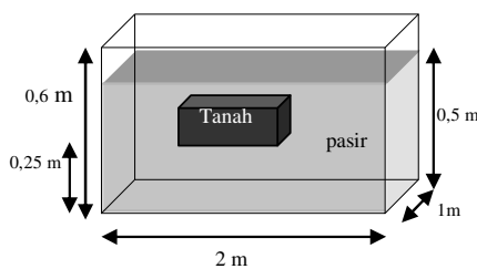
Gambar 5. Medium penelitian berupa pasir dan tanah liat
