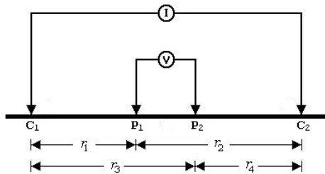
Gambar 1. Dua pasang elektroda arus dan potensial pada permukaan medium homogen isotropis dengan tahanan jenis \rho (Bahri, 2005)
