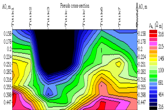
Gambar 7. Penampang isoresistivitas 2D setelah injeksi air pertama
