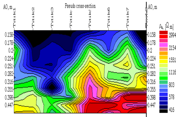
Gambar 10. Peta Isoresistivitas 2D setelah injeksi air keempat
