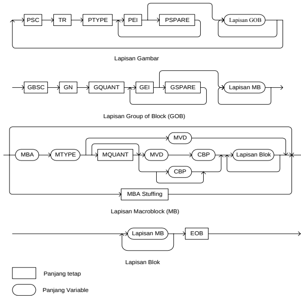
Gambar 2. Struktur aliran data video H.261 [1]
