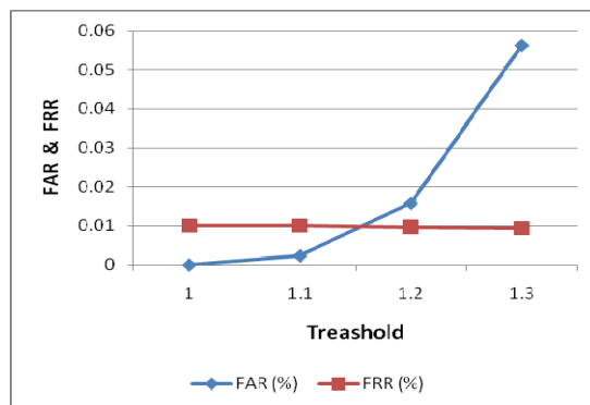
Gambar-5. Kurva Karakteristik 101 pengguna Menggunakan 10 eigenface
