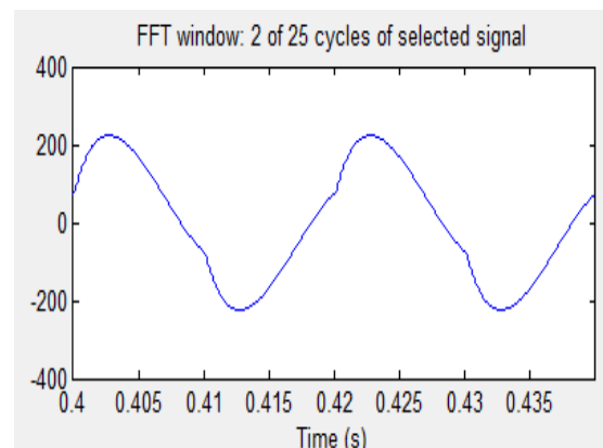
Gambar 3. Hasil Simulasi
