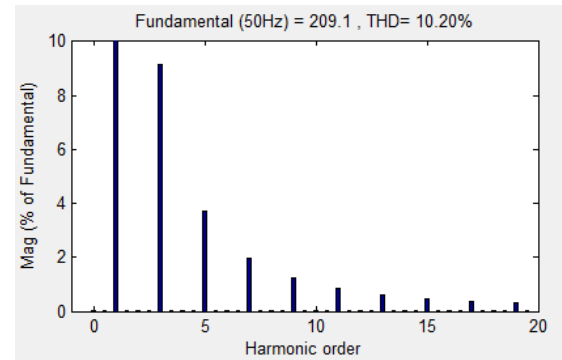
Gambar 4. Spektrum Harmonisa
