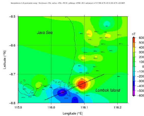
Gambar 1. Plot anomali geomagnetik 2D di Pulau Lombok (Zubaidah dkk., 2006)
