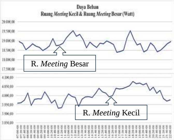
Gambar 9: Perbandingan Karakteristik Daya Penggunaan R. Meeting Besar & Kecil Secara Realtime
