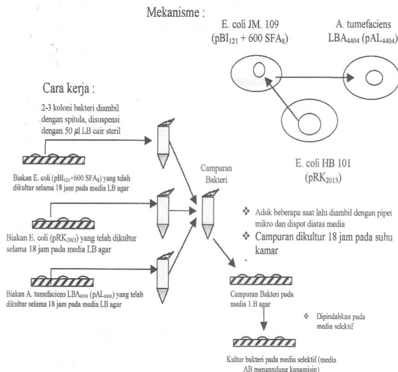
Gambar 1 : Skema kerja metode triparental mating
