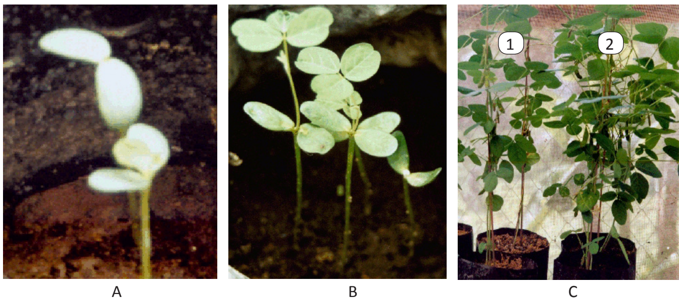
Gambar 3. Transformasi gen albumin secara in planta pada tanaman kedelai dengan vektor A. tumefaciens LBA 4404 . (A) Bibit kedelai diinokulasi pada bagian meristem di atas kotiledon. (B) Pertumbuhan tunas di atas kotiledon setelah ditransformasi. (C) Tanaman kedelai transgenik yang dihasilkan melalui transformasi in planta . 1. Kontrol (non transformed). 2. Tanaman transgenik dengan percabangan yang banyak, dibandingkan dengan kontrol
