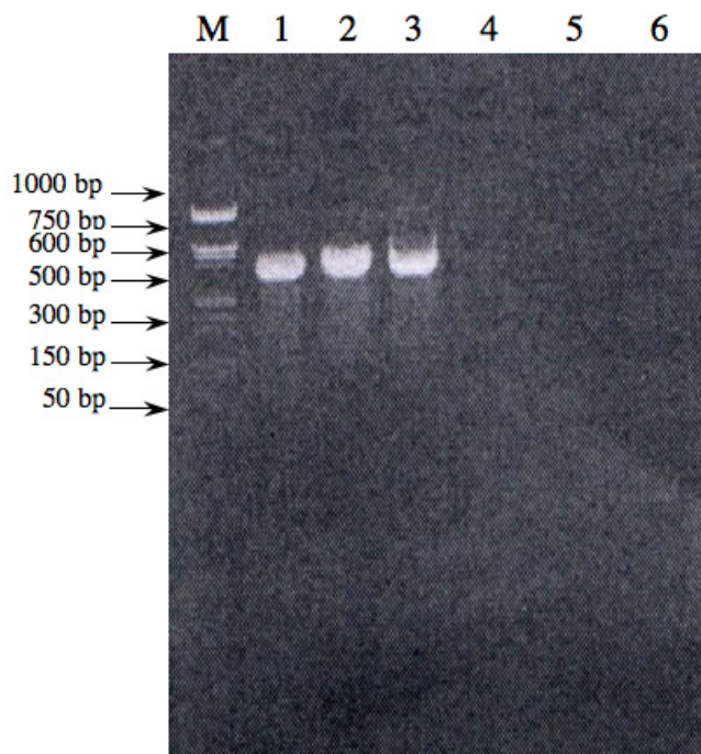
Gambar 4. Deteksi gen albumin bunga matahari pada tunas muda tanaman kedelai transgenik hasil transformasi. lane 1,2,3 merupakan kedelai transgenik dan lane 4,5,6 adalah kedelai non transgenik,, M = Marker
