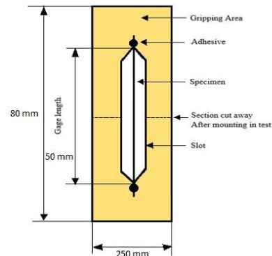
Gambar 1. Uji tarik serat tunggal
