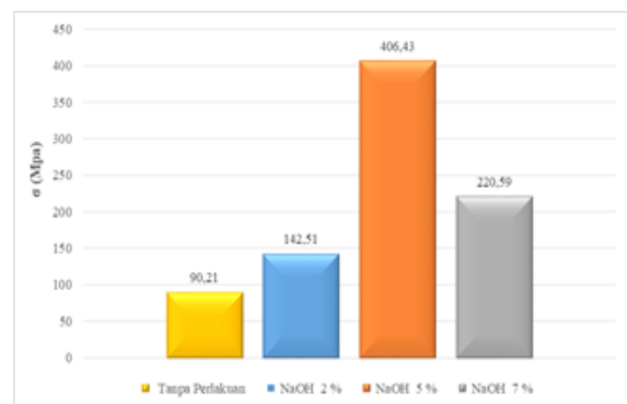
Gambar 4. Grafik Tegangan Tiap Perlakuan
