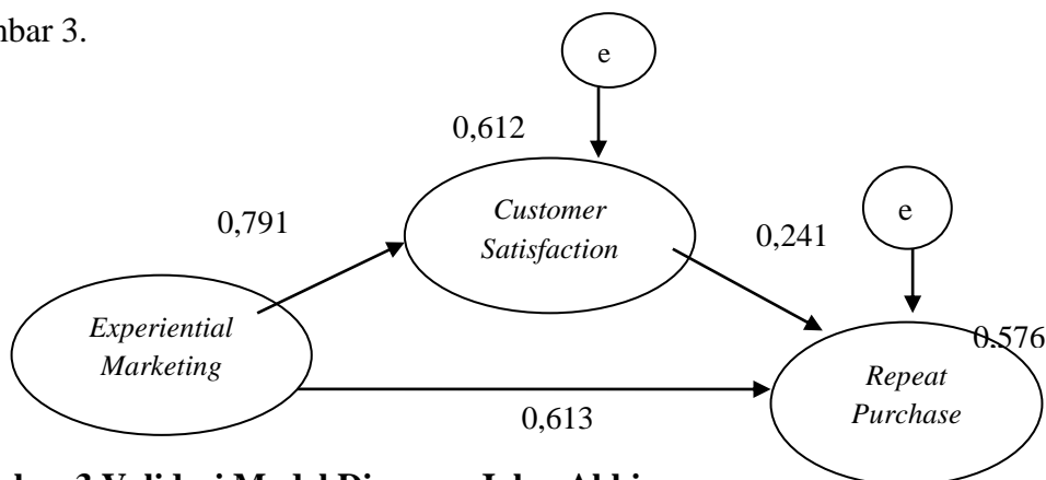
Gambar 3. Validasi Model Diagram Jalur Akhir
