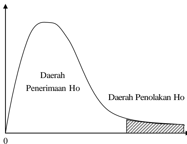
Gambar 1. Daerah Penolakan dan Penerimaan Ho dengan Uji F
