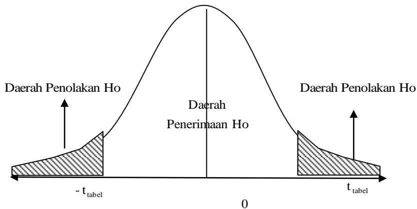
Gambar 2. daerah Penolakan dan Penerimaan H_0 dengan uji t
