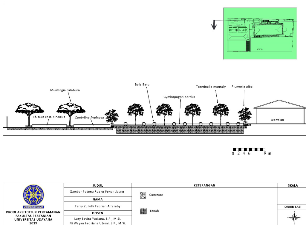
Gambar 2. Gambar Potong
