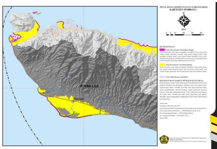
Gambar 2. Peta Zona Kerentanan Likuefaksi di Kabupaten Jembrana Sumber Gambar: Atlas Zona Kerentanan Likuefaksi Indonesia, Badan Geologi Kemen ESDM,
