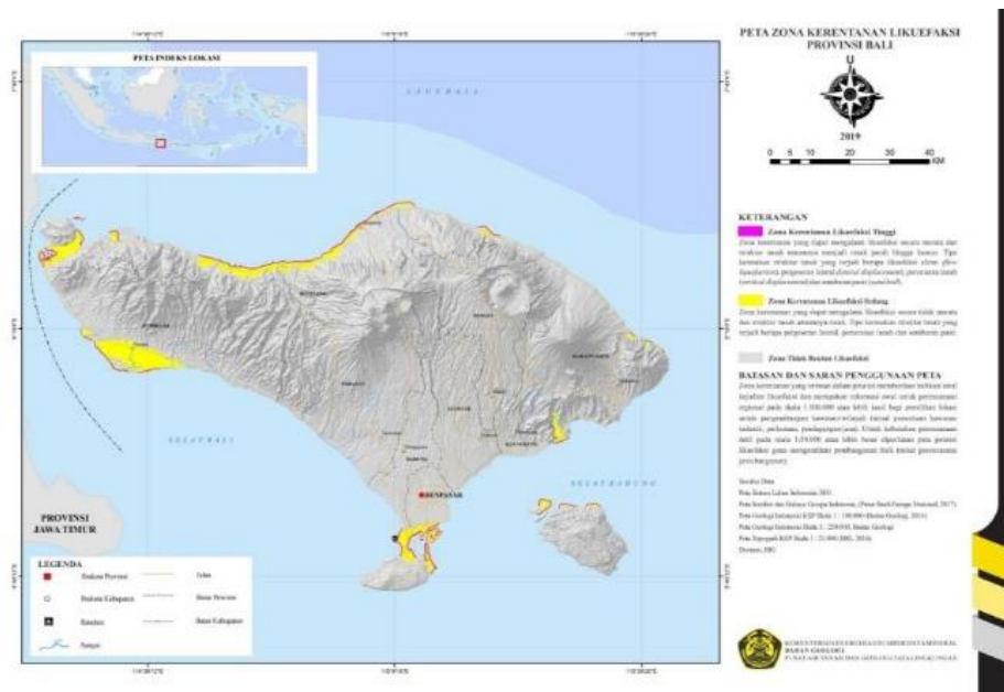
Gambar 1. Peta Zona Kerentanan Likuifaksi di Provinsi Bali
