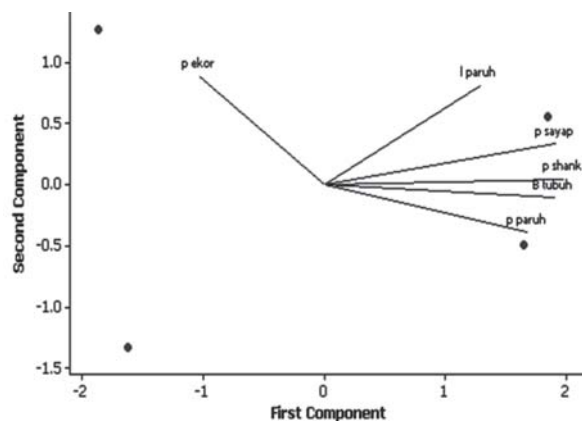
Gambar 2 Proyeksi karakter morfologi untuk empat lokasi dalam bidang dua dimensi.
