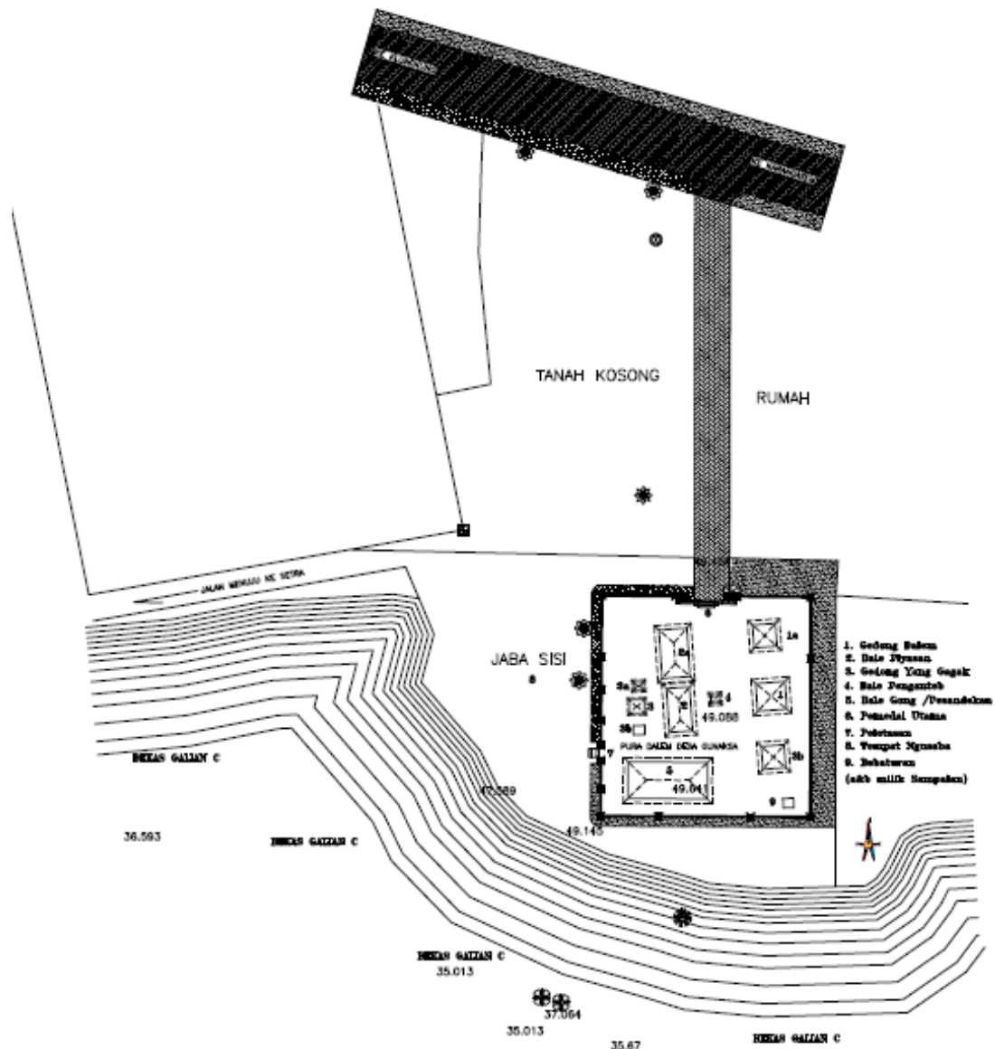
Gambar 3.1. Lay Out Lingkungan Pura Dalem Desa Gunaksa
