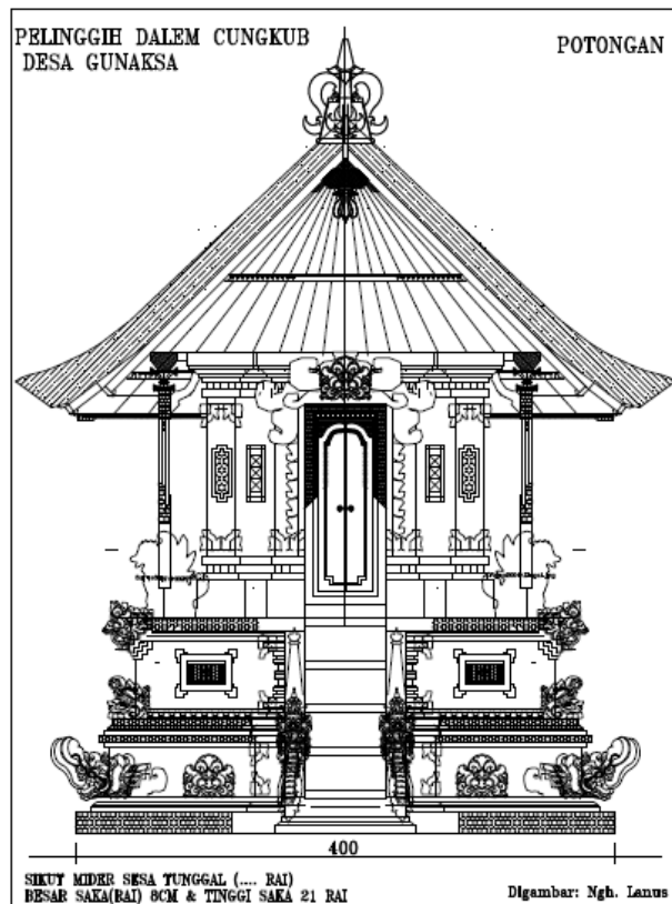
Gambar 3.3.Potongan Palinggih Gedong Pura Dalem Desa Gunaksa
