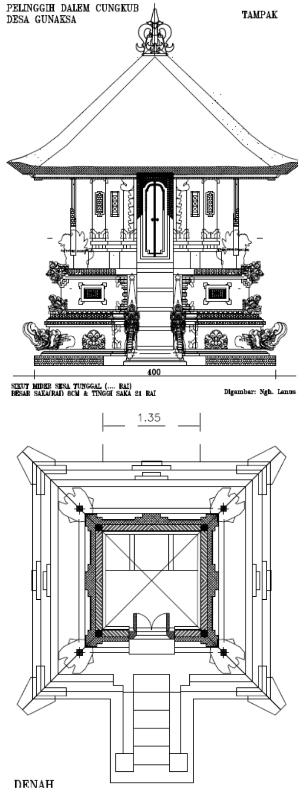
Gambar 3.2. Denah dan Tampak Palinggih Gedong Pura Dalem Desa Gunaksa
