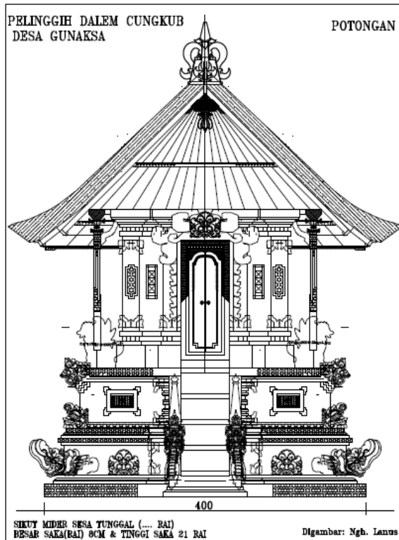
Gambar 3.3.Potongan Palinggih Gedong Pura Dalem Desa Gunaksa
