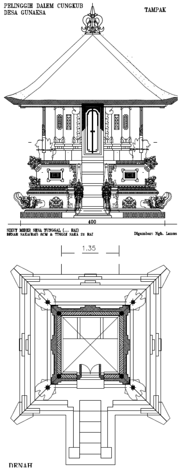
Gambar 3.2. Denah dan Tampak Palingih Gedong Pura Dalem Desa Gunaksa
