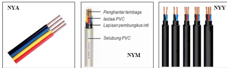
Gambar 2.5. Jenis kabel Arus Kuat
