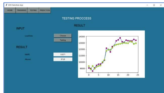
Gambar 5. Hasil prediksi
