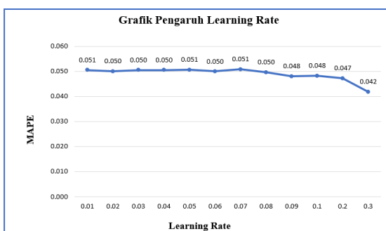
Gambar 4. Pengaruh learning rate terhadap MAPE
