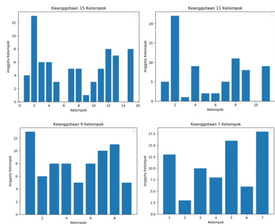
Gambar 2. Keanggotaan Kelompok
