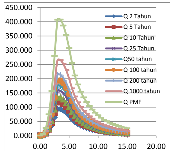
Gambar 5 Gambar grafik hidrograf Nakayasu
