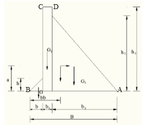
Gambar 2 Gaya-gaya vertikal pada tubuh bendungan (Sumber: Soedibyo, 2003)
