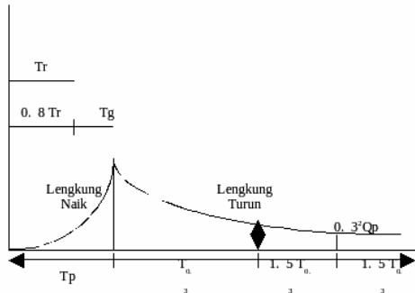
Gambar 1 Hidrograf satuan sintetik Nakayasu (Sumber: Sri Harto, 1993)
