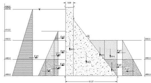
Gambar 7 gambar gaya-gaya yang terjadi pada tubuh bendungan
