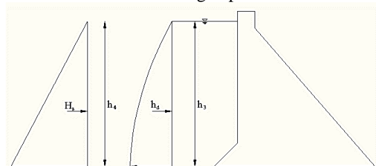
Gambar 3 Gaya-gaya horizontal pada tubuh bendungan (Sumber: Soedibyo, 2003)
