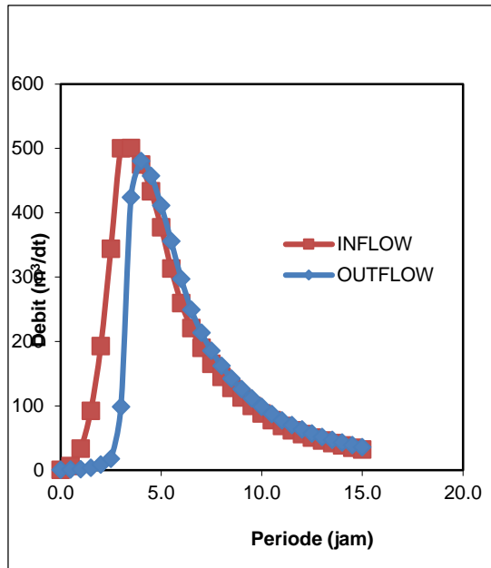
Gambar 6 gambar grafik hubungan waktu dengan debit
