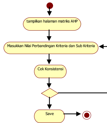
Activity Diagram Kelola Matriks Kriteria dan Sub
