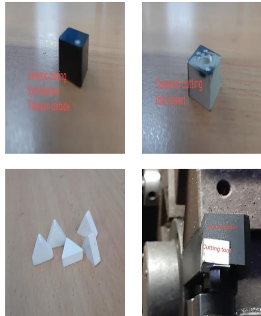
Gambar.3 Mata Pahat Keramik
