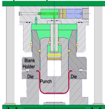
Gambar 2. Bagian Utama Die Drawing
