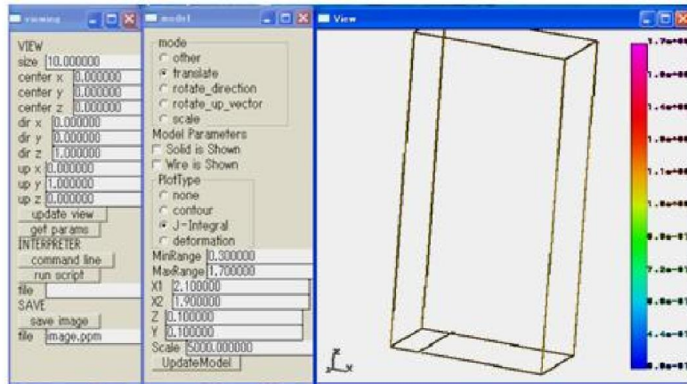
Gambar 4 Visualisasi model beserta retakannya
