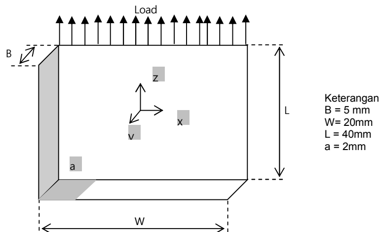
Gambar 3 Pemodelan untuk analisa retakan
