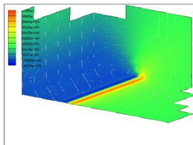
Gambar 6 \sigma_z pada puncak retakan
