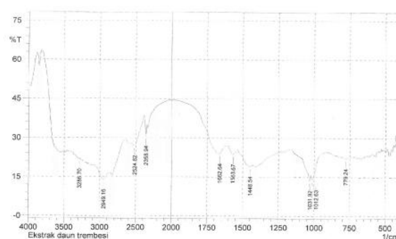
Gambar 3. Spektrum inframerah hasil identifikasi isolat B
