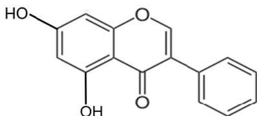
Gambar 5. Struktur 5,7 dihidroksi isoflavon
