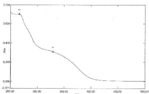
Gambar 4. Spektrum UV-Vis dari isolat B
