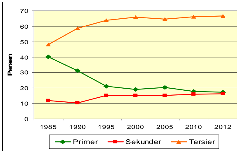
Gambar 3 Kontribusi Sektor Primer, Sekunder dan Tersier Terhadap PDRB Provinsi Bali, 1985 – 2012
