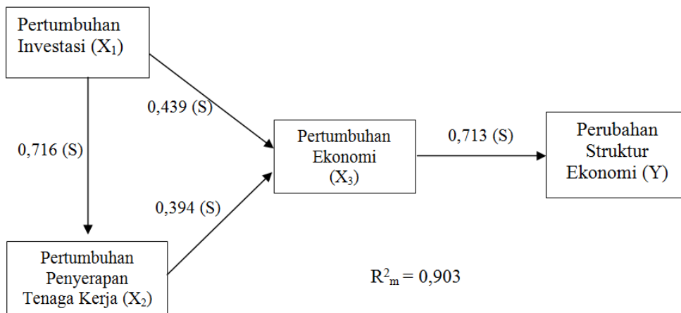
Gambar 6 Diagram Jalur Pengaruh Variabel Pertumbuhan Investasi, Pertumbuhan Penyerapan Tenaga Kerja dan Pertumbuhan Ekonomi Terhadap Perubahan Struktur Ekonomi (Setelah Dimodifikasi)
