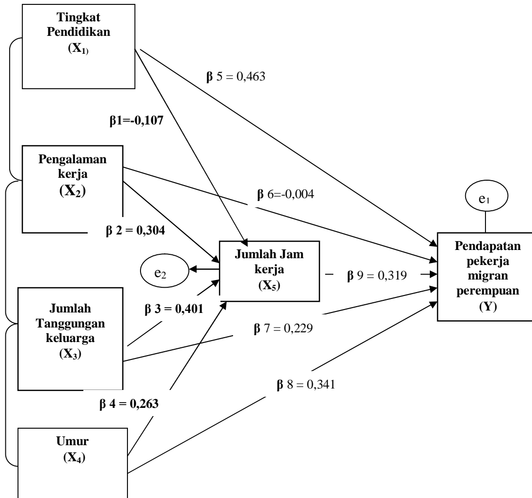
Gambar 1. Koefisien Jalur
