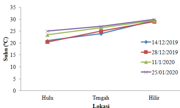
Gambar 4. Grafik Nilai Suhu dari Hulu ke Hilir
