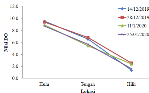
Gambar 2. Grafik Penurunan DO dari Hulu ke Hilir
