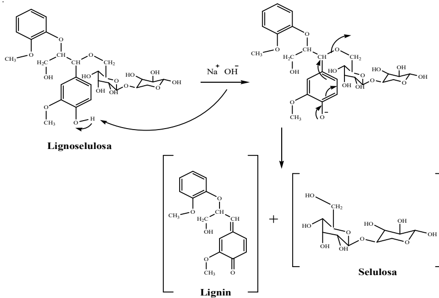
Gambar 1. Mekanisme reaksi pemutusan ikatan lignin dan selulosa
