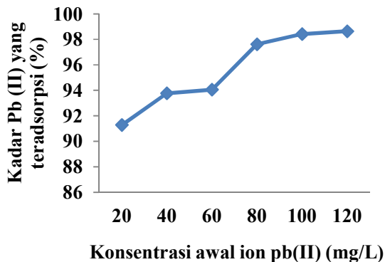
Gambar 7. Persentase logam Pb yang terserap oleh adsorben cangkang buah karet
