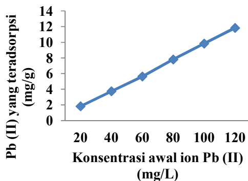
Gambar 6. Grafik pengaruh konsentrasi awal larutan Pb
