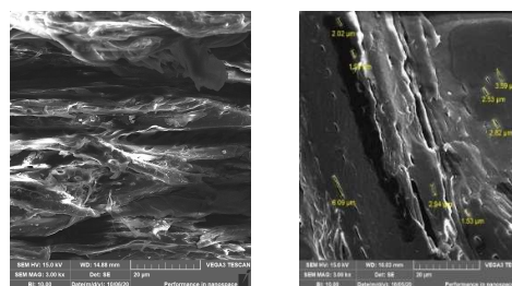
Gambar 4. Adsorben sebelum delignifikasi (a) dan adsorben setelah delignifikasi (b)
