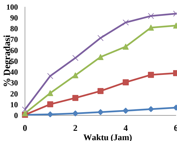
Gambar 5. Pengaruh waktu irradiasi terhadap persentase degradasi (%D) dari larutan Rhodamin B 100 ppm pada sistem yang berbeda. \blacklozenge : sistem I ( \text{ZnO/pH} optimum tanpa penyinaran) ; \blacksquare : sistem II ( \text{ZnO/UV/pH} optimum); \blacktriangle : sistem III ( \text{ZnO/UV/H}_2\text{O}_2/\text{pH} optimum); \times : sistem IV ( \text{ZnO/UV/H}_2\text{O}_2/\text{Fe}^{2+}/\text{pH} optimum).
