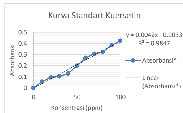
Gambar 2. Kurva Standar Kuersetin
