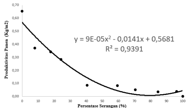
Gambar 4. Grafik Analisis Regresi Kuadrat
