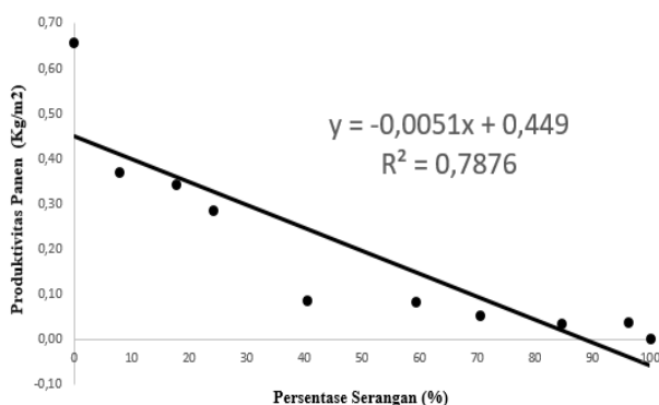
Gambar 3. Grafik Analisis Regresi Linier
