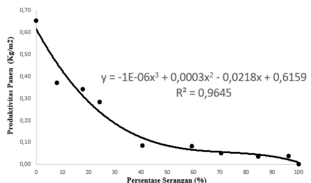
Gambar 5. Grafik Analisis Regresi Polinomial
