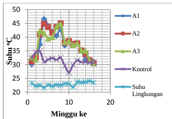
Gambar 1. Suhu di bagian tengah tumpukan.
