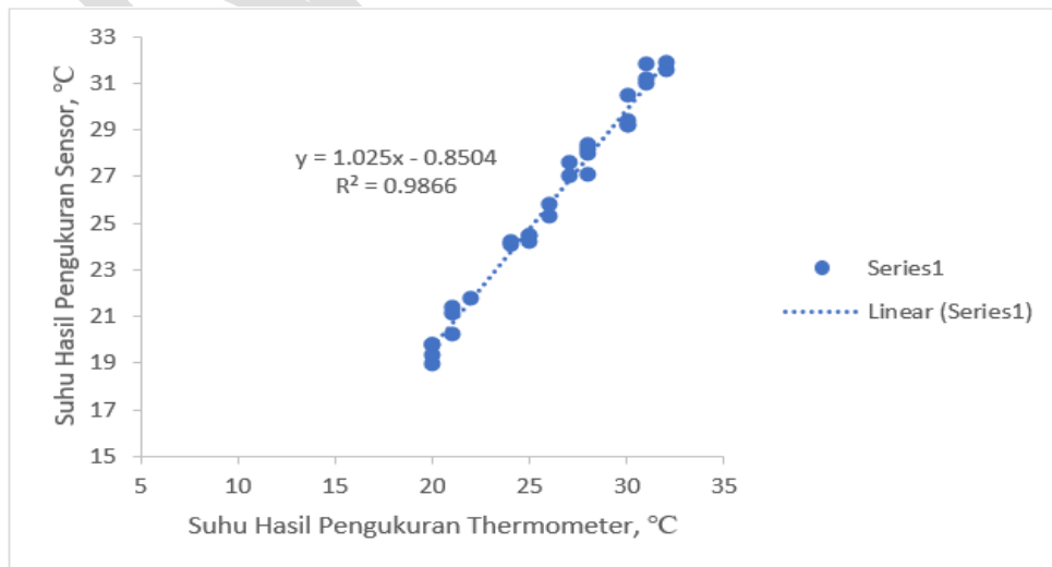
Gambar 3. Hubungan dan Suhu dari Kedua Hasil Pengukuran
