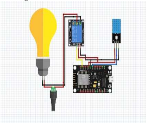
Gambar 2. Skema Rangkaian Alat
