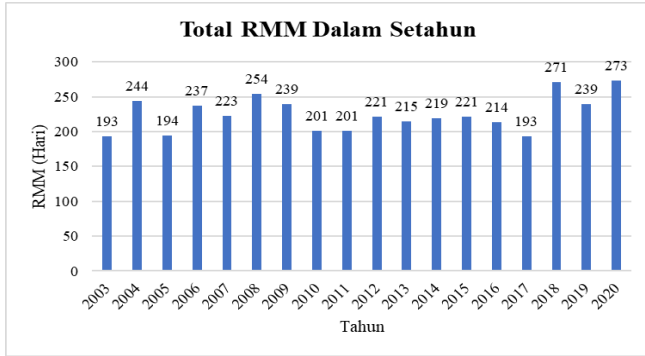
Gambar 2. Total RMM dalam Setahun
