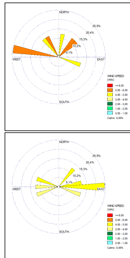
Gambar 8. Windrose Wilayah F (atas) dan Wilayah G (bawah)
