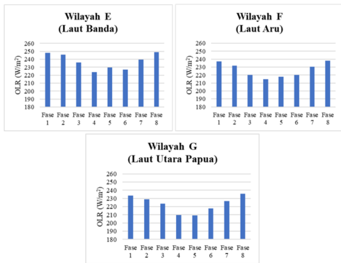
Gambar 4. Grafik OLR Wilayah A – Wilayah G
