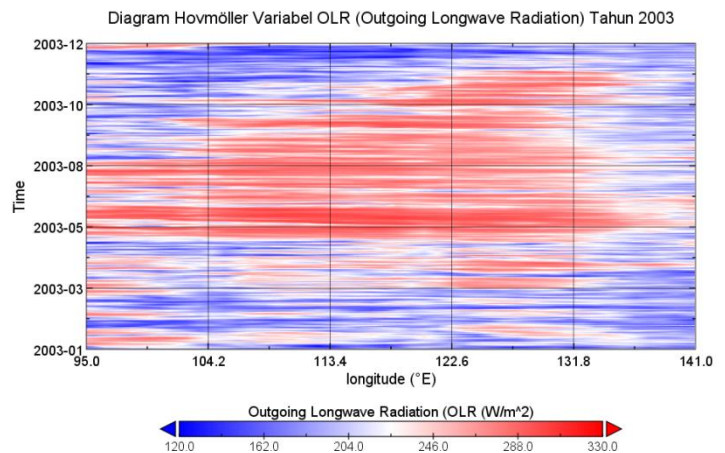
Gambar 5. Diagram Hovmöller Variabel OLR Tahun 2003
