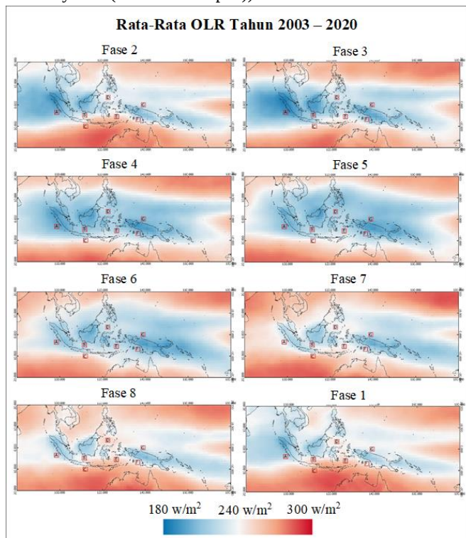
Gambar 3. Pergerakan MJO Berdasarkan Rata-Rata OLR Tahun 2003 – 2020
