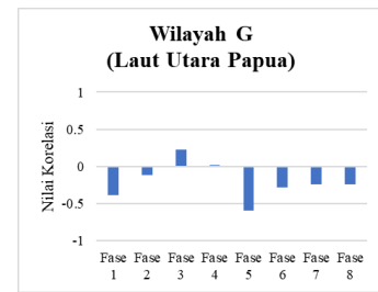
Gambar 7. Grafik Hubungan OLR dengan Kecepatan Angin Wilayah A – Wilayah G Tahun 2003 – 2020
