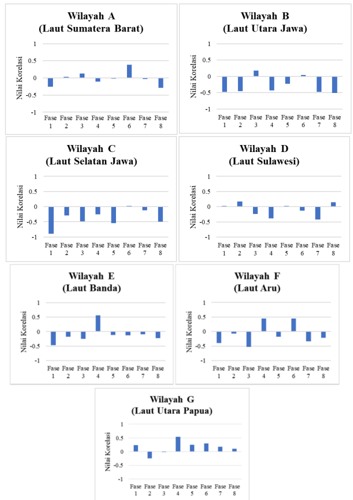
Gambar 9. Grafik Hubungan OLR dengan SPL Wilayah A – Wilayah G Tahun 2003 – 2020
