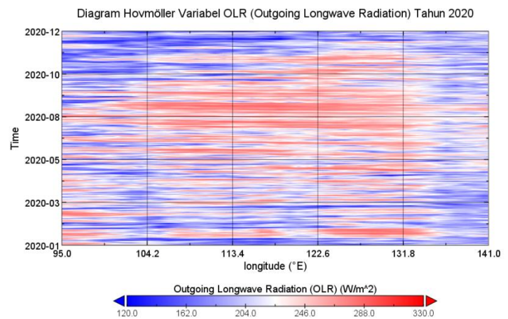
Gambar 6. Diagram Hovmöller Variabel OLR Tahun 2020
