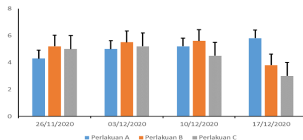
Gambar 2. Pertumbuhan Batang Seledri ( A. graveolens )
