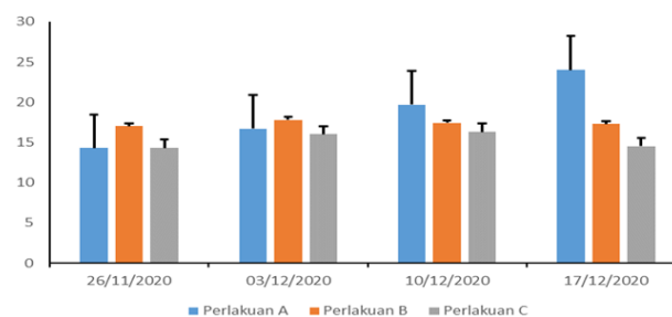
Gambar 3. Pertumbuhan Daun Seledri ( A. graveolens )
