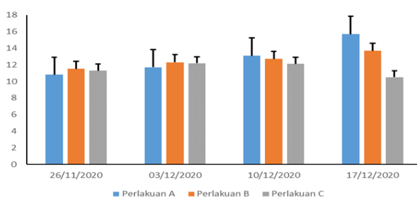
Gambar 1. Pertumbuhan Tinggi Seledri ( A. graveolens )
