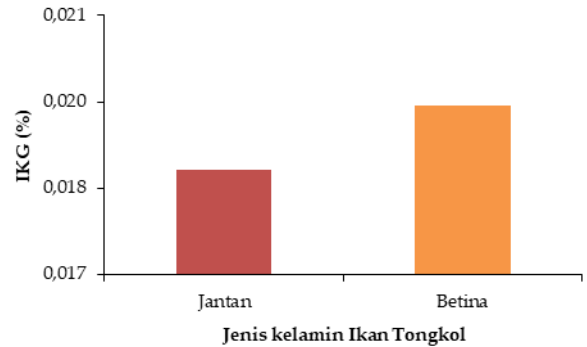
Gambar 4. Indeks Kematangan Gonad Ikan Tongkol di Perairan Kusamba
